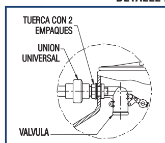
DETALLE 2
