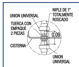
DETALLE 2
