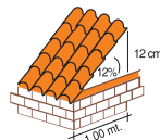
Pendiente Mínima 7° (12%)
